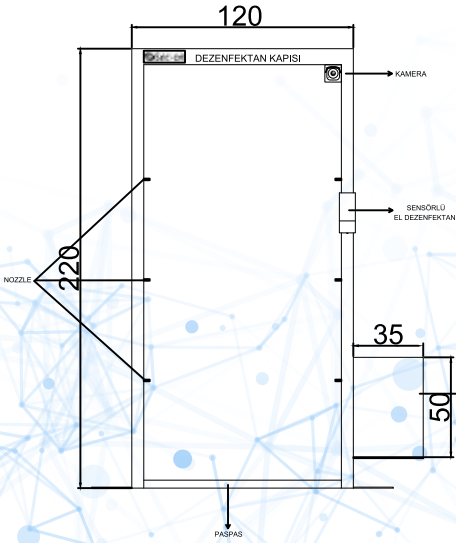
ÖNDEN GÖRÜNÜŞ
